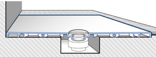
MONTAJE A RAS
