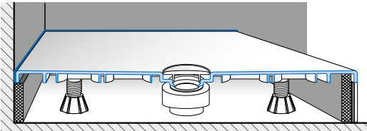
MONTAJE SOBRE ZÓCALO
