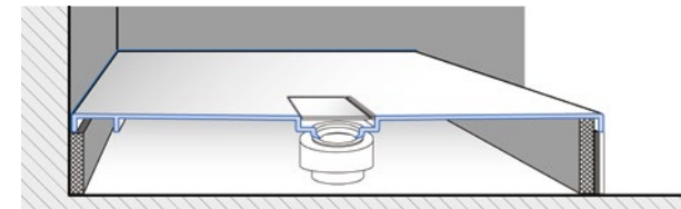
MONTAJE SOBRE ZÓCALO
