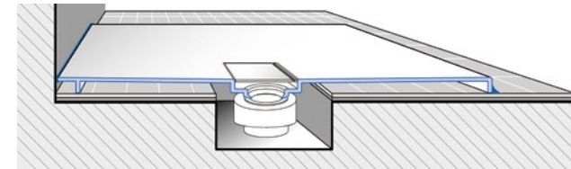
MONTAJE SOBRE BALDOSAS
