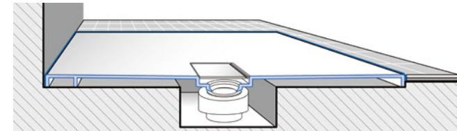
MONTAJE A RAS
